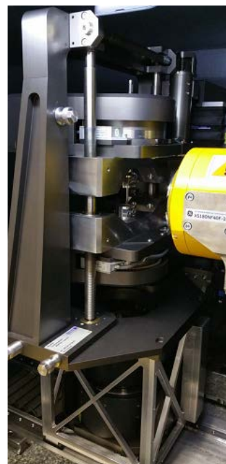
Prüfung mit der CT-insitu-Belastungsprüfvorrichtung (Torsion: Schulterzugprobe)
